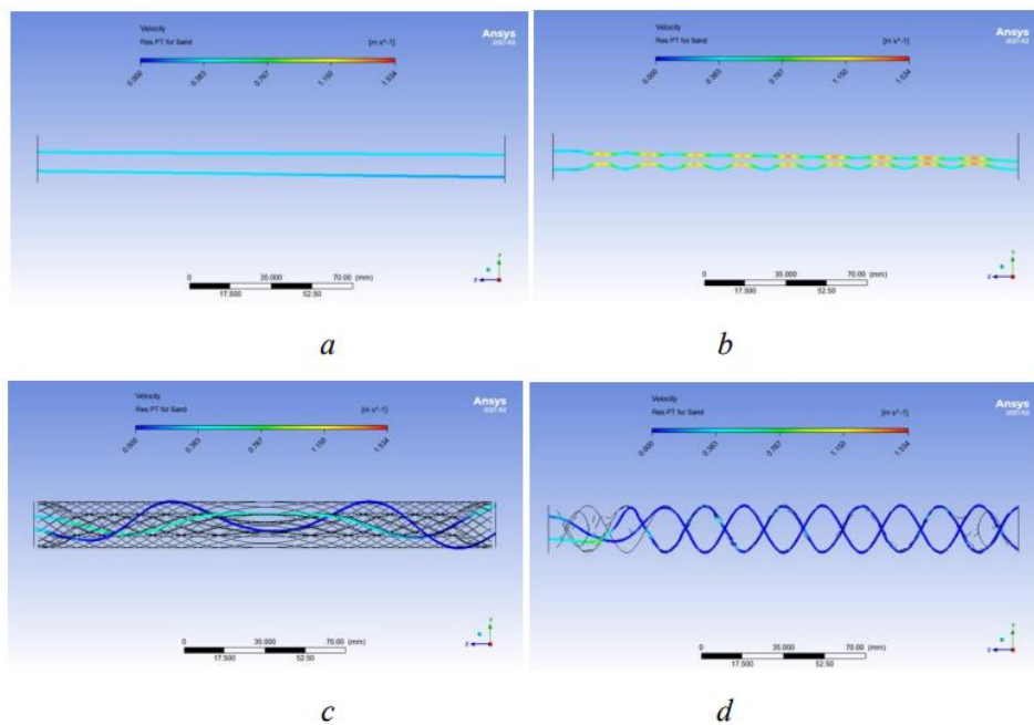
Рис. 2. Траєкторія швидкості точок рідини в трубі: а - круглий переріз, б - сферичний переріз, с - зірко-реверсивний переріз, д - спіральний переріз.
