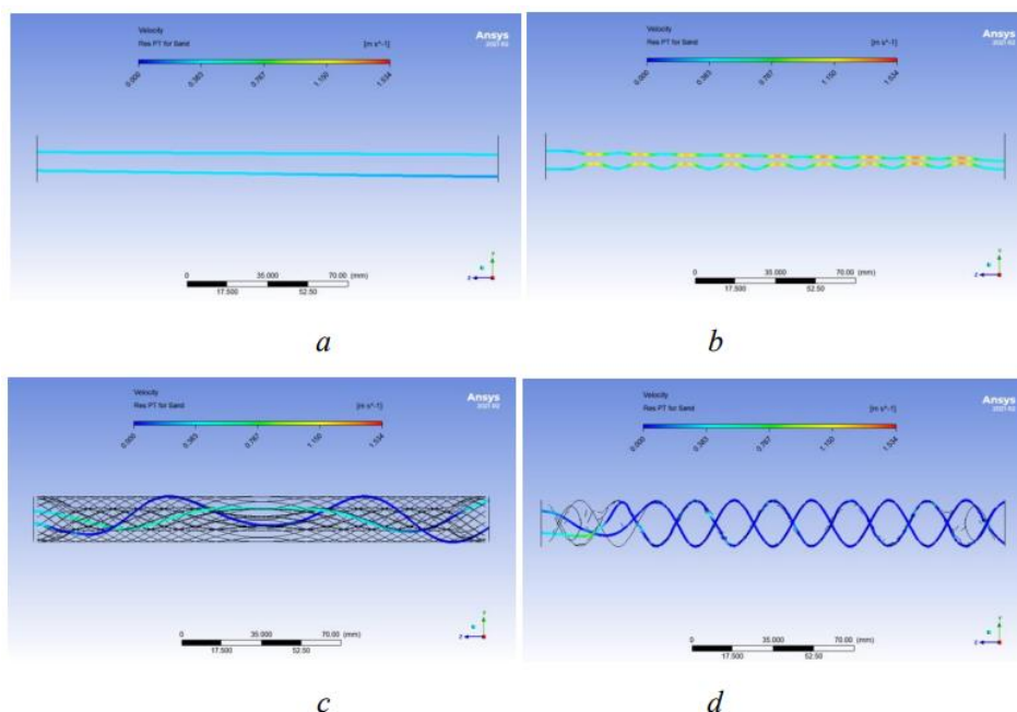
Рис. 2. Траєкторія швидкості точок рідини в трубі: а - круглий переріз, б - сферичний переріз, с - зірко-реверсивний переріз, d - спіральний переріз.
